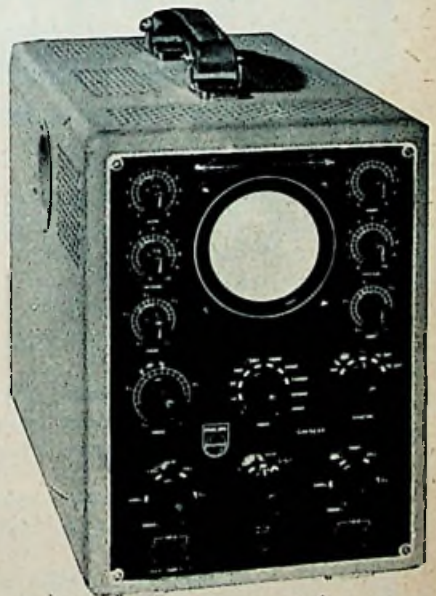
Philips electronoscillograaf G. M. 5659
